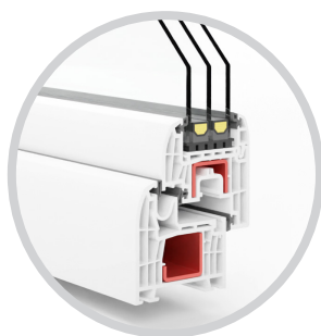
T-Classic Slim 27 % mehr Licht 7 Kammern Uw 0,85 W/m²K
