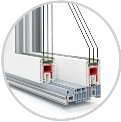
Schwelle 50 mm richtet sich nach dem Bodenniveau aus
